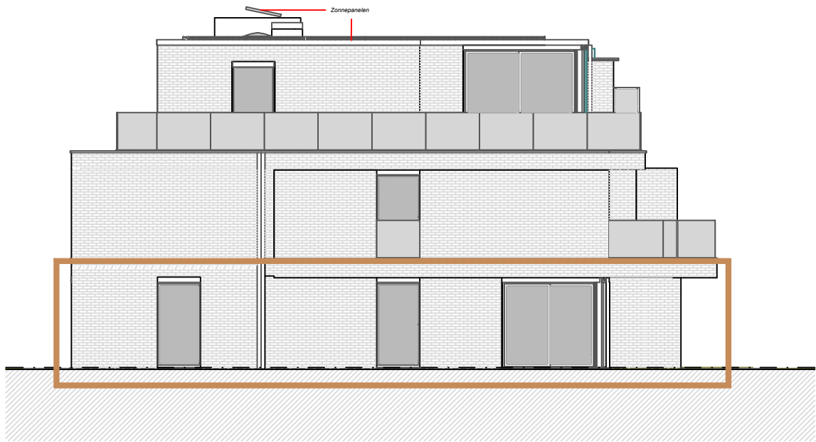
ZIJGEVEL WEST
