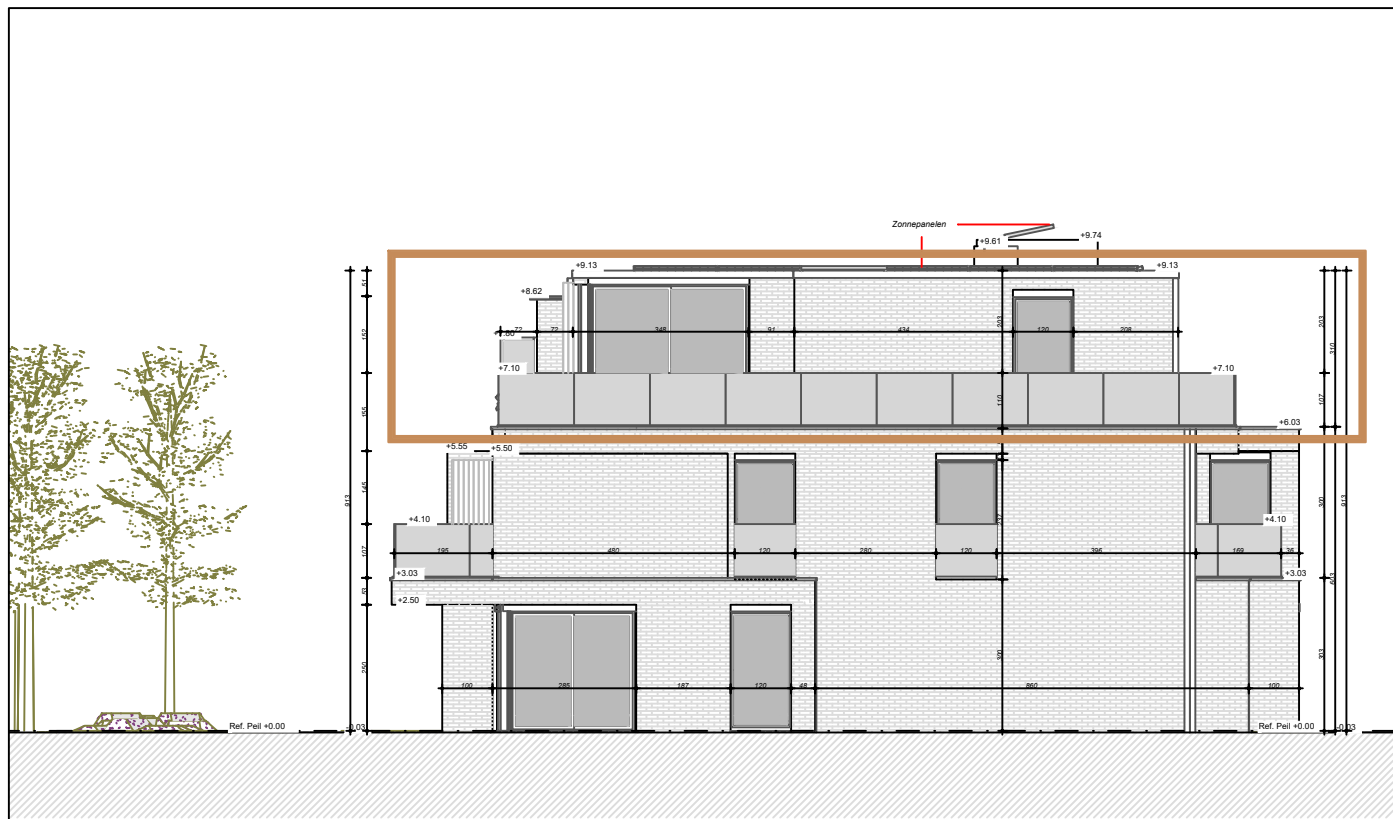
ZIJGEVEL (OOST)
